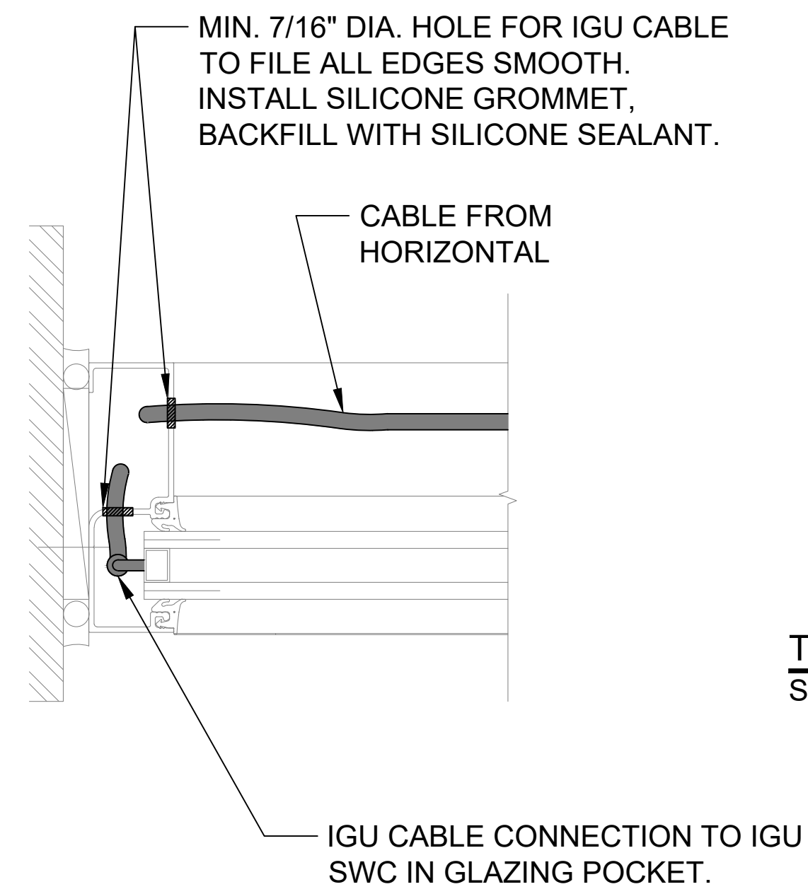
DETAIL 4 LEFT JAMB
